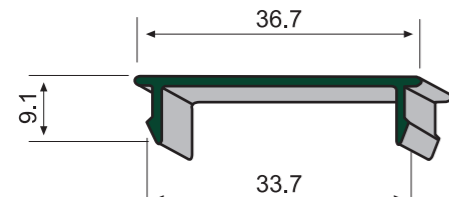
B/ 806 Grapa de la U B502
