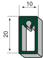
B/ 812 Rectangular de 20 x 10 auto
