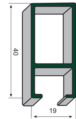
C/ 307P Perfil soporte cristal
