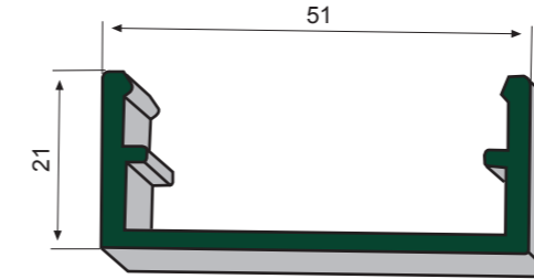
B/ 102 U de barandilla cristal
